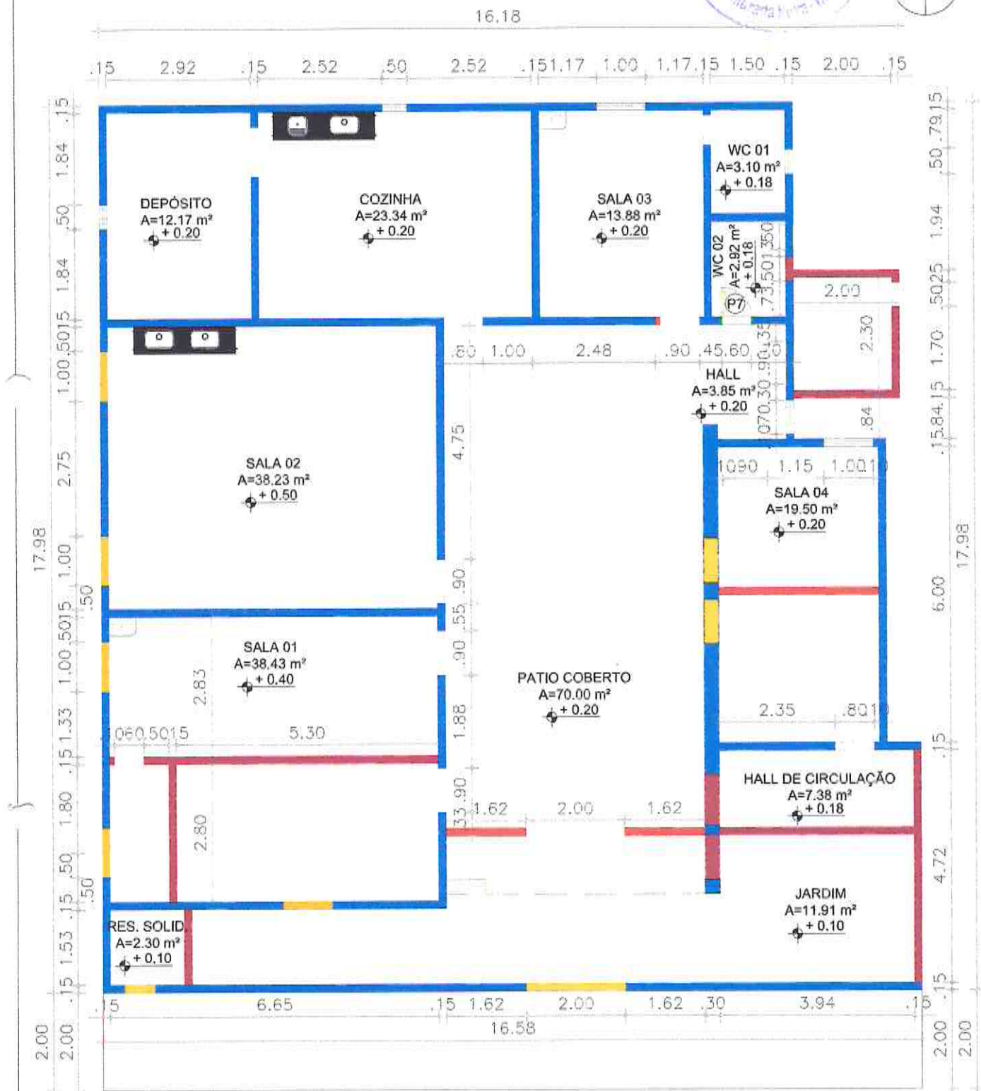
1 Planta baixa demolir construir Escala 1/100
