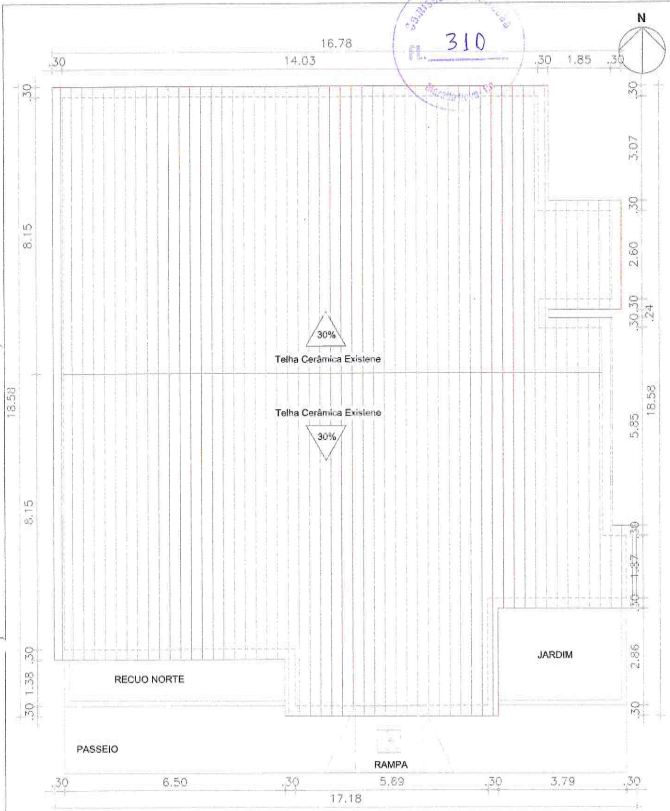
1 Planta de cobertura Escala 1/100
