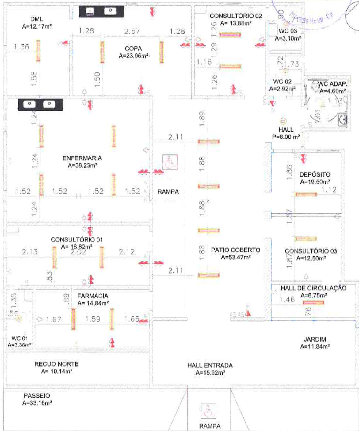
1 Planta Baixa pontos elétricos Escala 1/100
