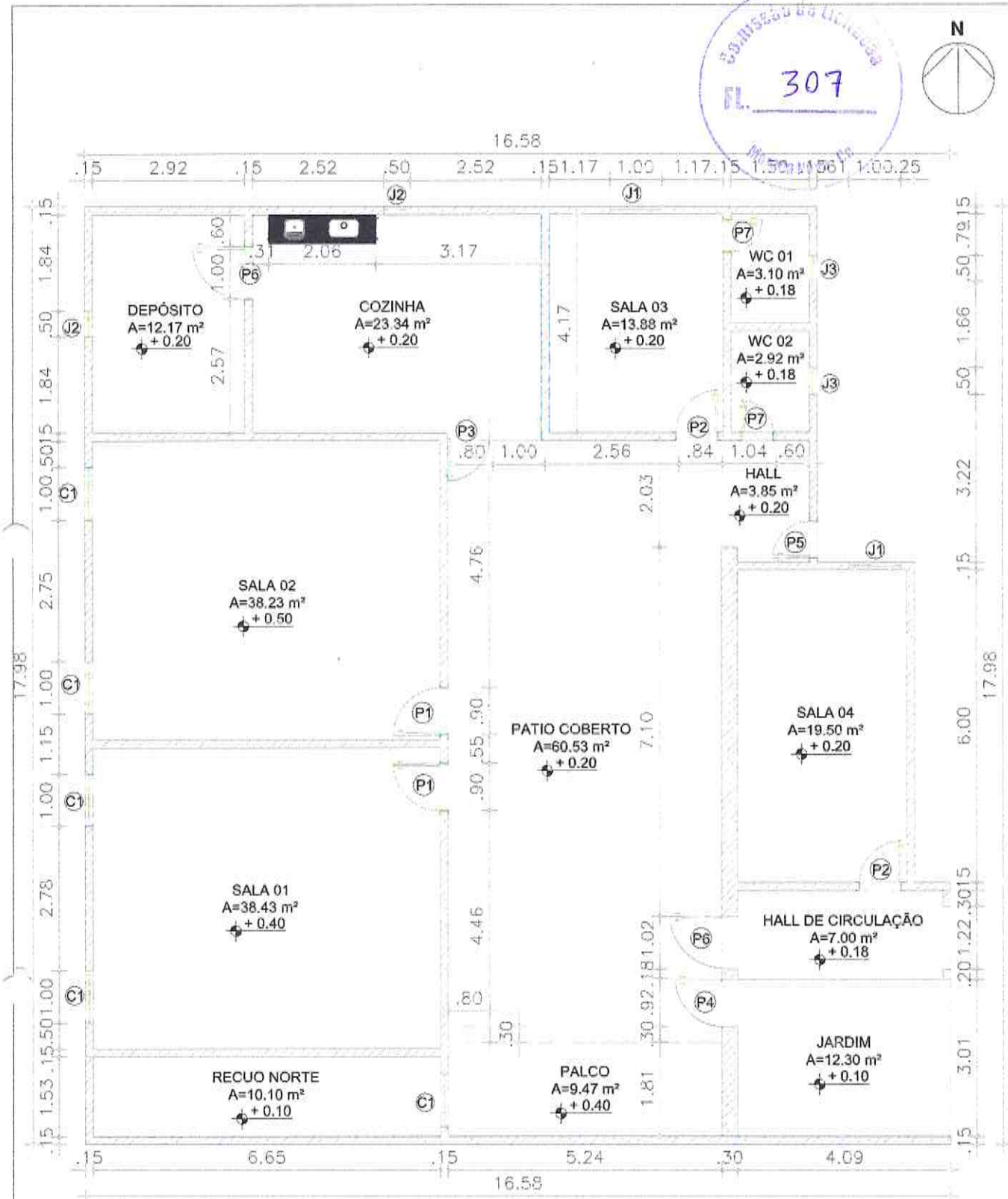
1 Planta Baixa de levantamento Escala 1/100
