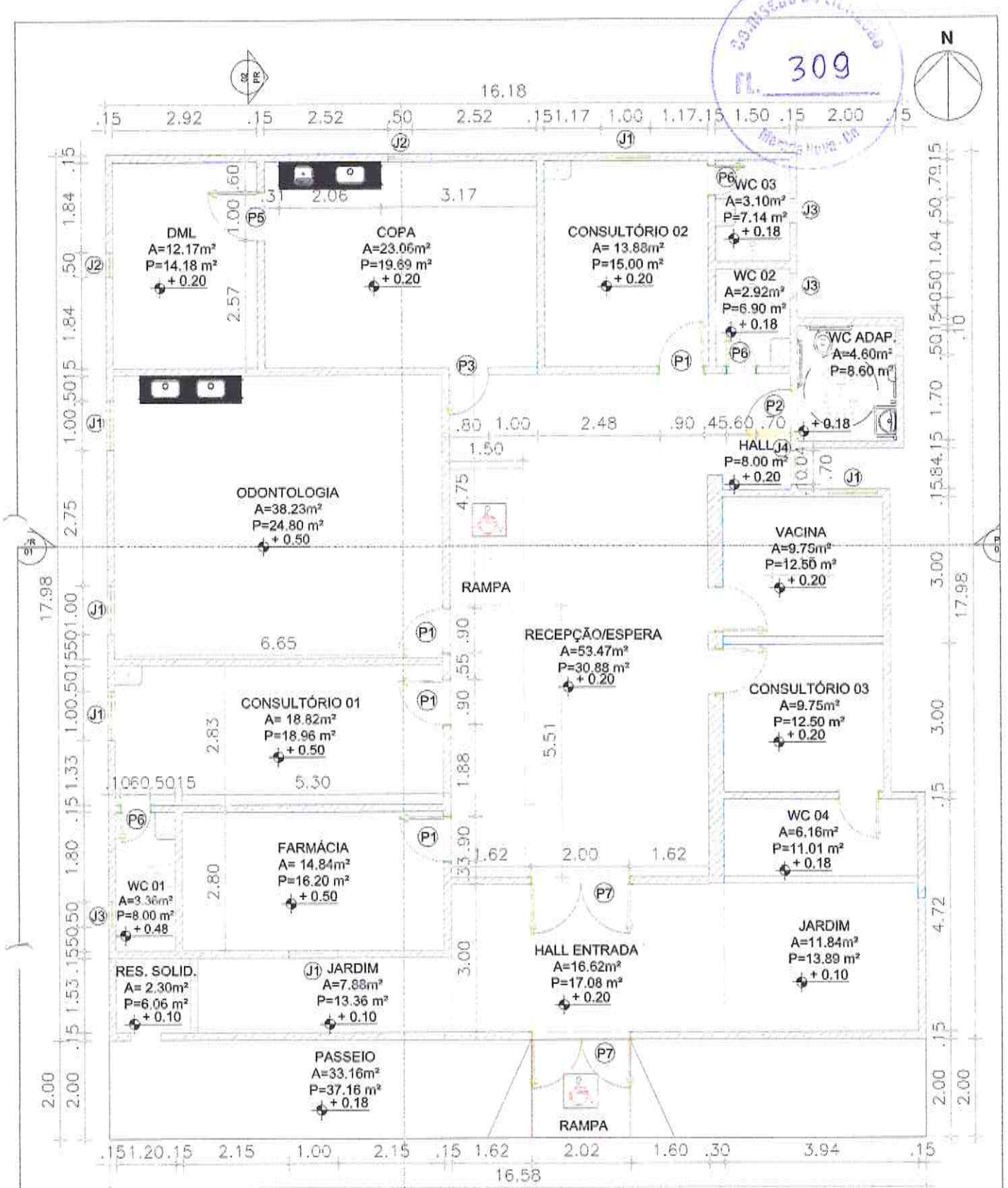
1 Planta Baixa atualizada Escala 1/100
