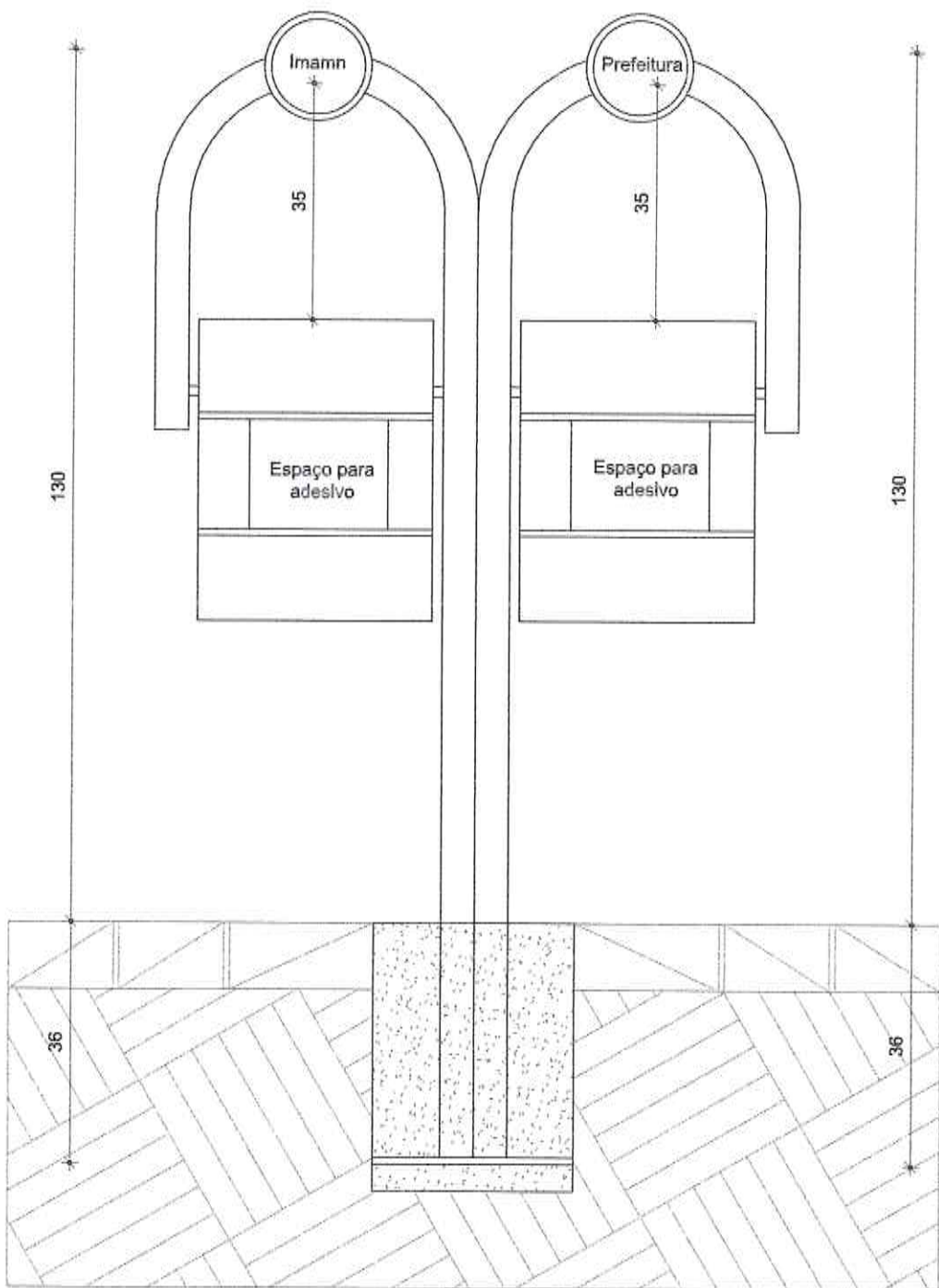
1 Corte Esquemático Escala 1/10
