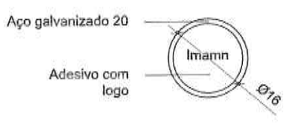
② Detalhe Escala 1/10
