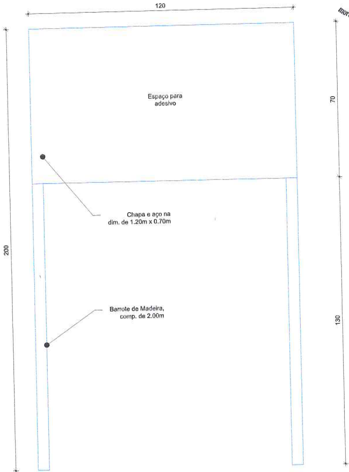
① Detalhe da Placa Escala 1/10
