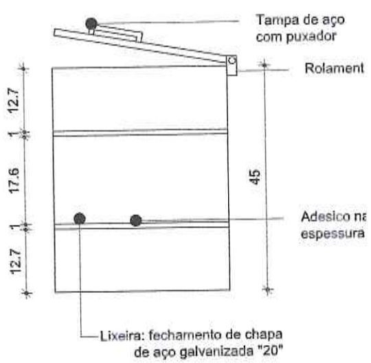
② Det. da Lixeira - Vista Frontal Escala 1/10
