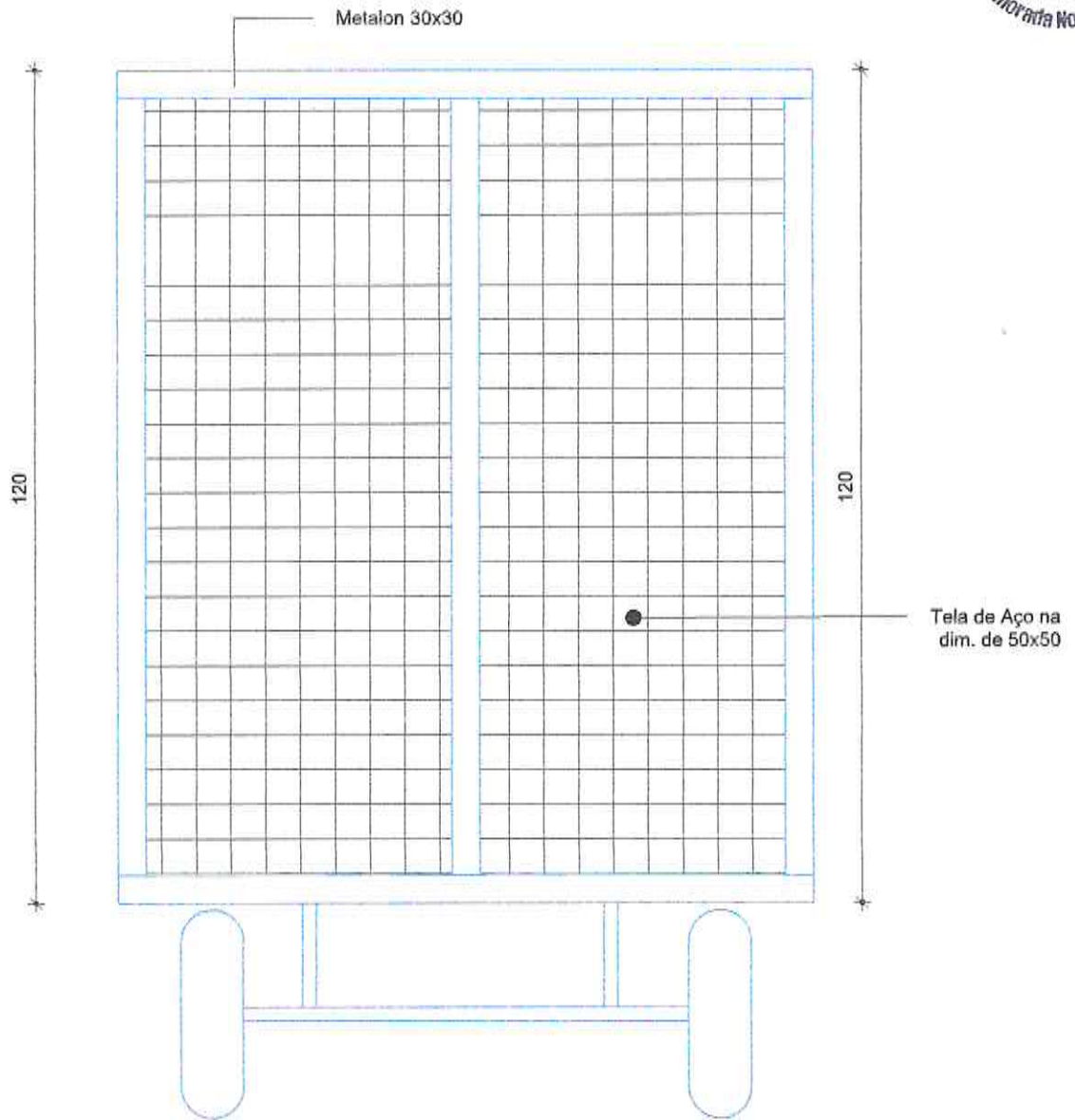
① Vista Posterior do Carrinho Escala 1/10
