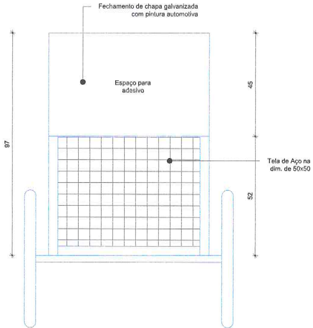
① Vista Posterior da Carreta Escala 1/10
