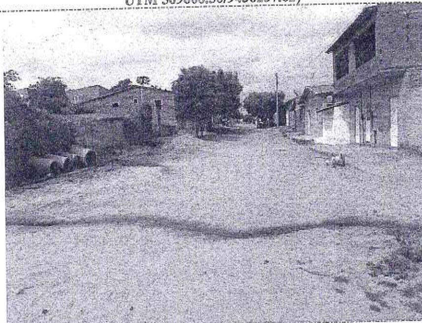
Final (Estaca E13 + 7,57m) do Trecho da Rua Luiz Damasceno Girão (Bairro: São Francisco) (Coordenada UTM 569641.04/9436356.39)
